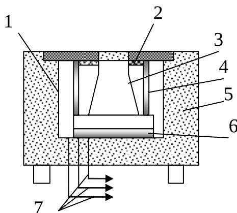
1 – циліндричний нагрівач; 2 – нагрівач горла реакційної колби; 3 – реакційна колба; 4 – елемент нагрівача; 5 – теплоізоляція; 6 – нагрівач дна; 7 – термодатчики
